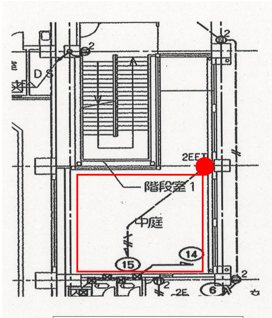
コンセント図
