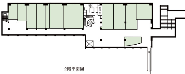
各階配置図
